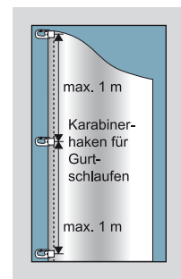
Hisselement unten
